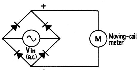
Fig. 2 Meter Rectifier.
